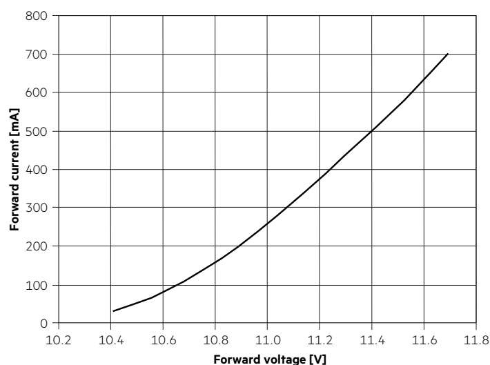
LLE 16x140mm 650lm 9xx HV ADV6
